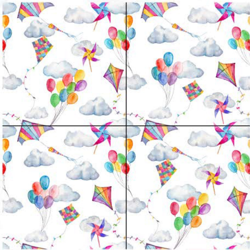
KC 018 (RANDOM)
